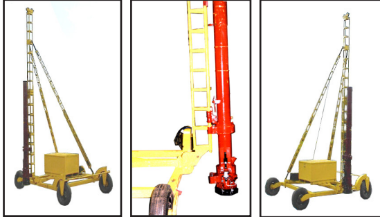
Complete mini-rig.
